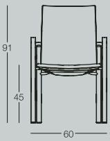
HIGH SILLÓN · ARMCHAIR
